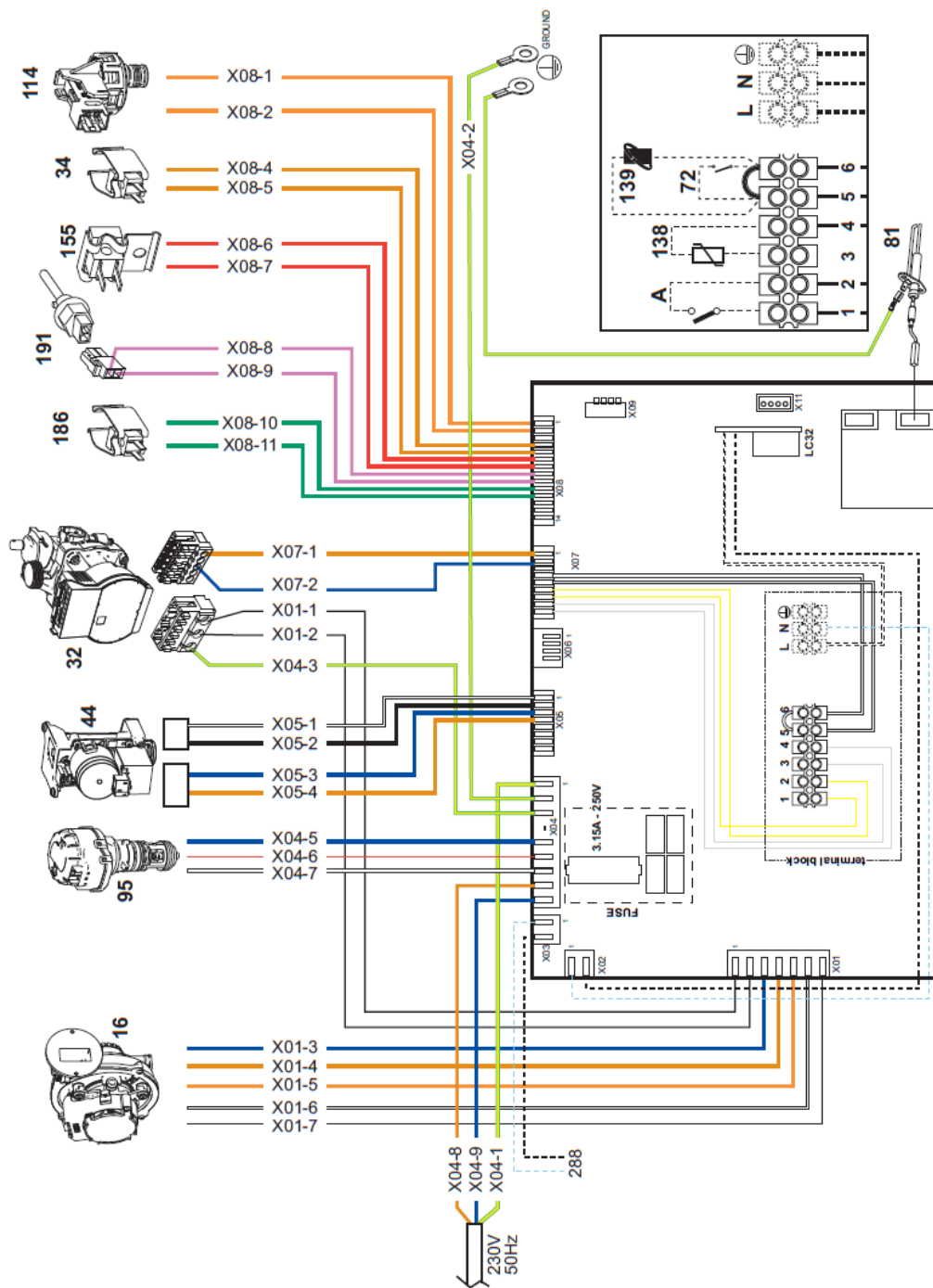
Rys. 43 Schemat instalacji elektrycznej
