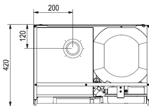
Rys. 36- Widok z góry
