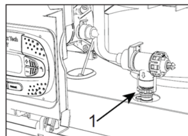
Rys. 17- Zawór bezpieczeństwa z kurkiem spustowym
