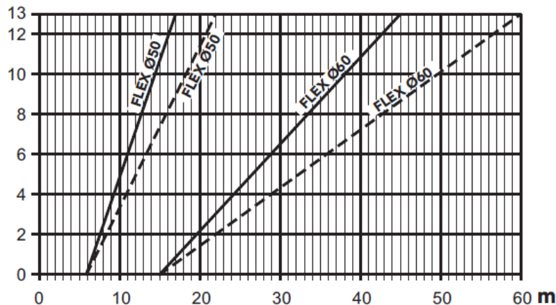
Rys. 26- Tabela wyboru parametrów przewodu spalinowego
