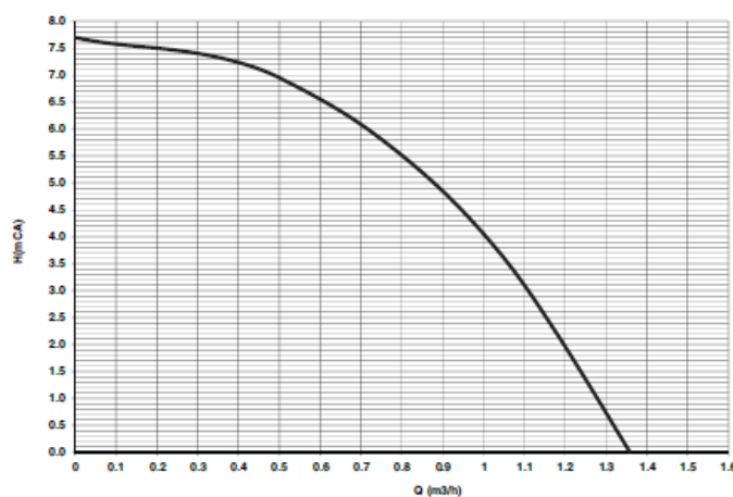
Rys. 41- Wysokość podnoszenia dostępna dla układu
