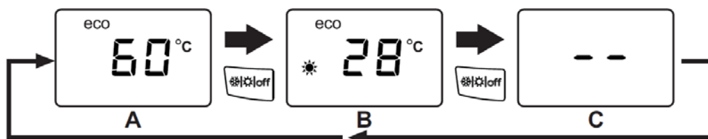
Rys. 8- Wyłączenie kotła
