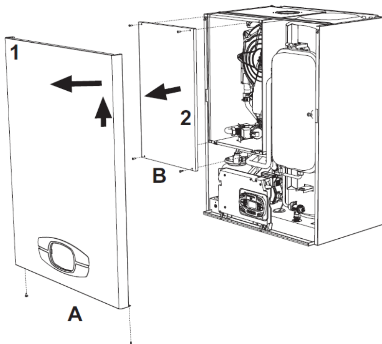
Rys. 32- Otwieranie panelu przedniego
