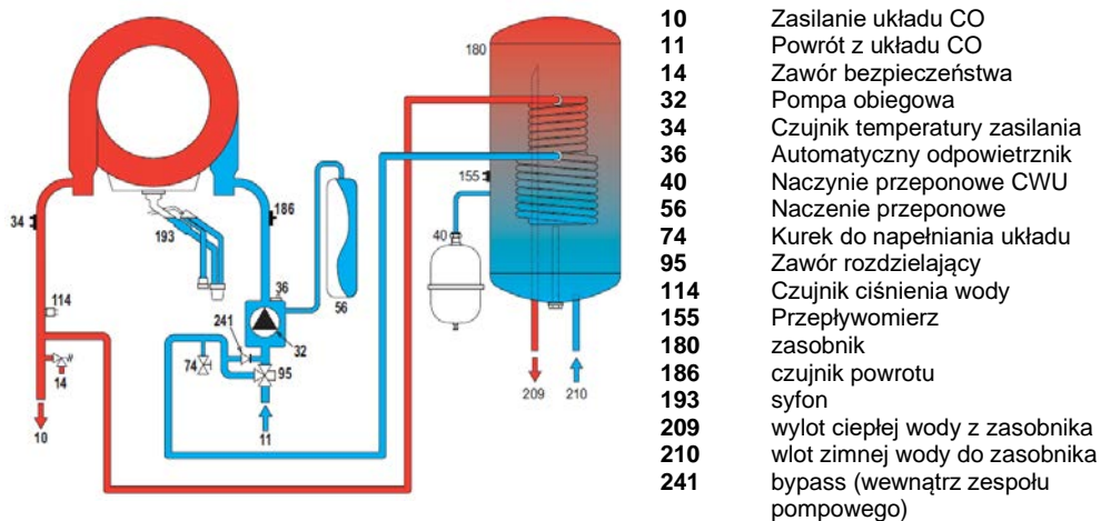
Rys. 39- Obieg wody
