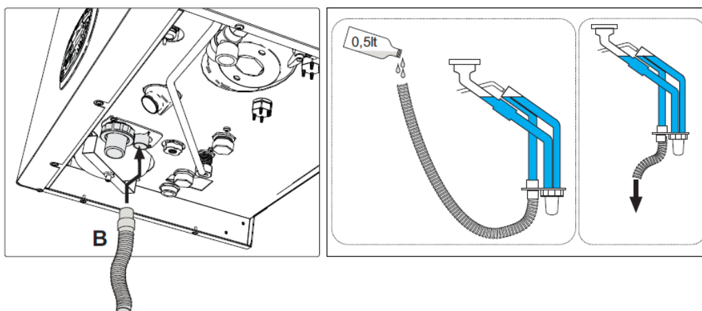
Rys. 29- Przyłącze spustowe kondensatu
