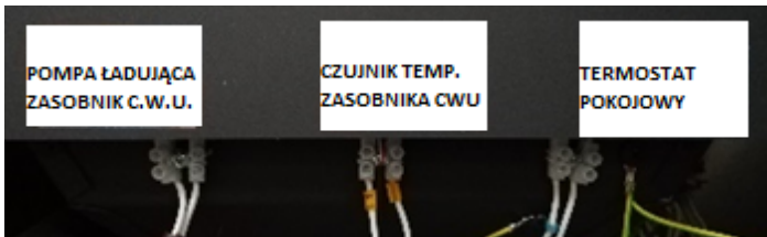
Zdjęcie listwy zaciskowej z tyłu urządzenia
