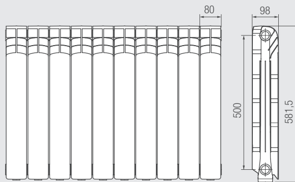
PROTEO 600 HP
