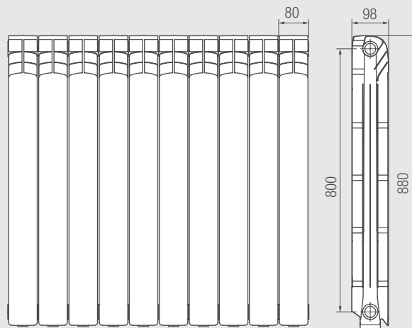
PROTEO 900
